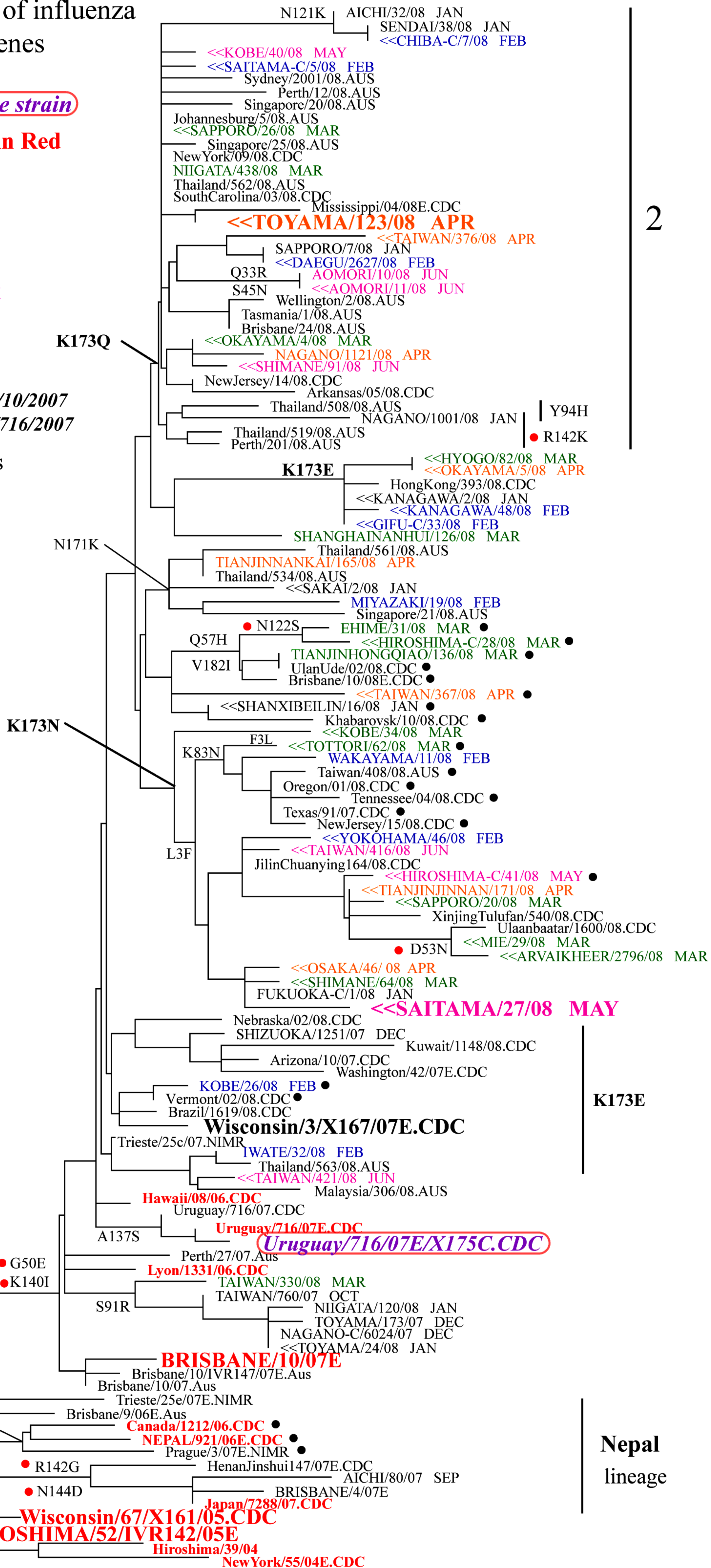
図 5. A/H3N2 ウイルス HA 遺伝子の系統樹解析
